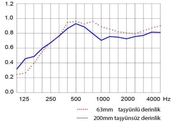
EN ISO 354 ses yutum katsayısı ölçümü
